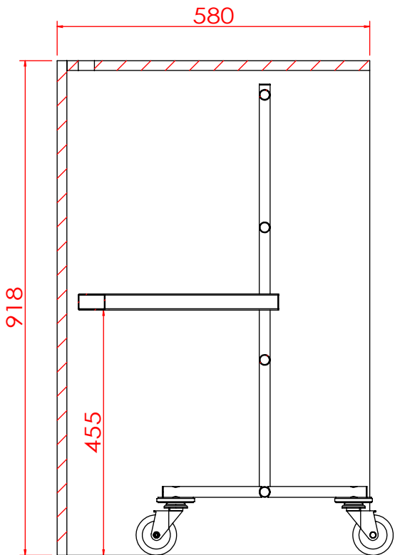
剖面 A-A
