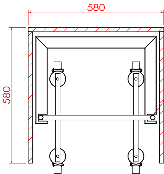
剖面 B-B
