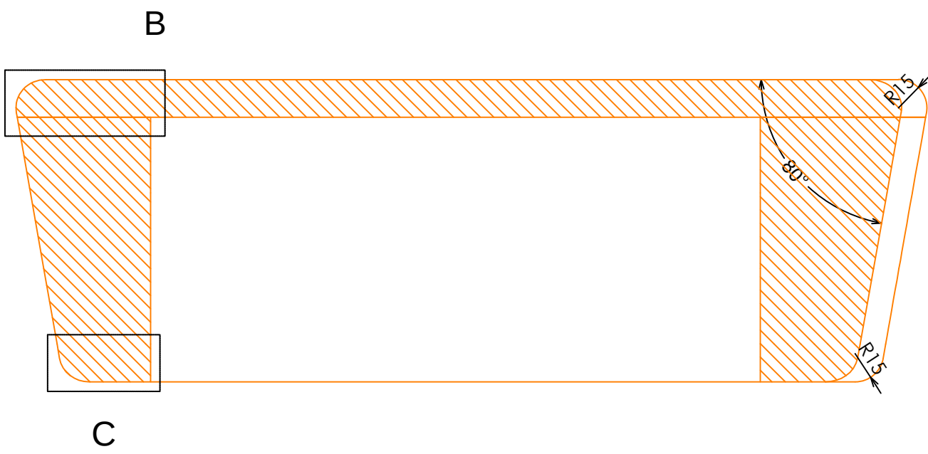
SECCIÓN A-A
