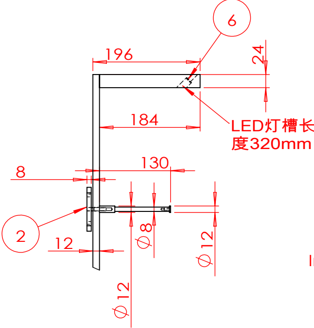
局部视图 C 比例 1 : 7
