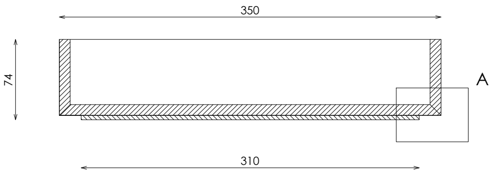
SECCION
