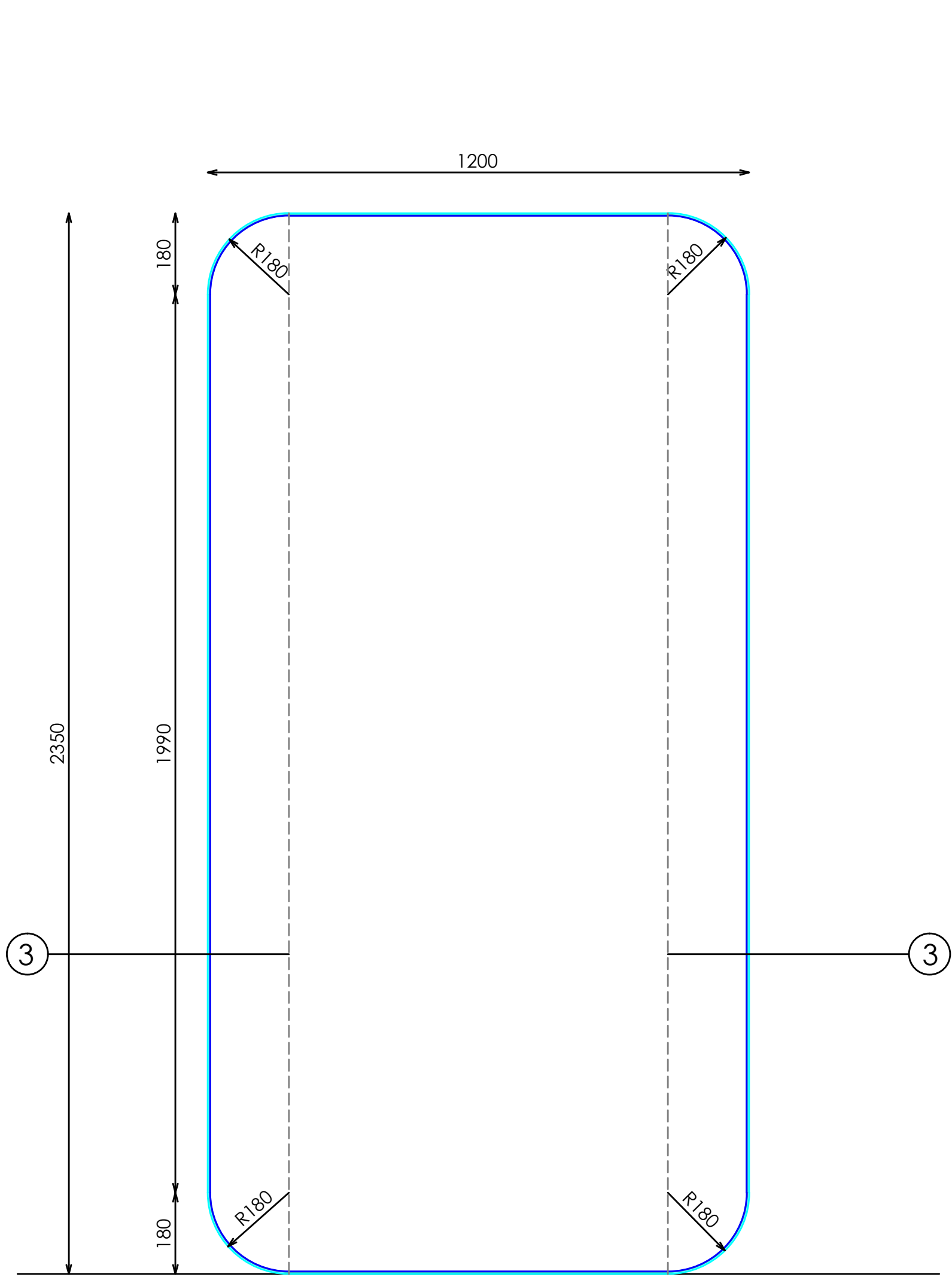
ALZADO
