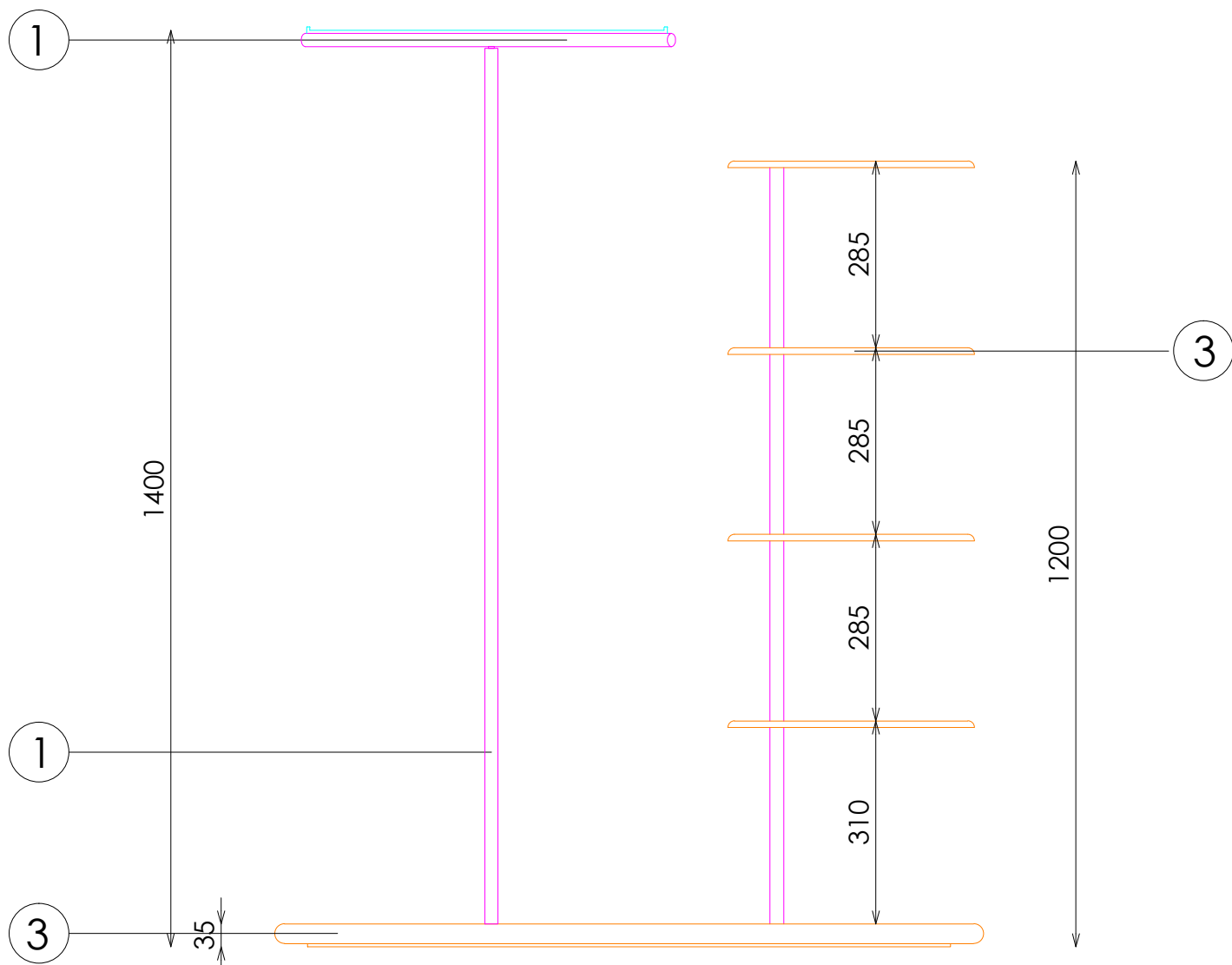
PERFIL DERECHO
