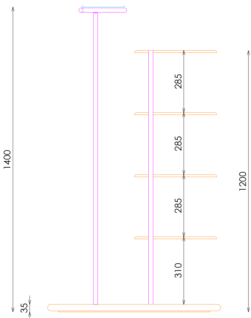
ALZADO
