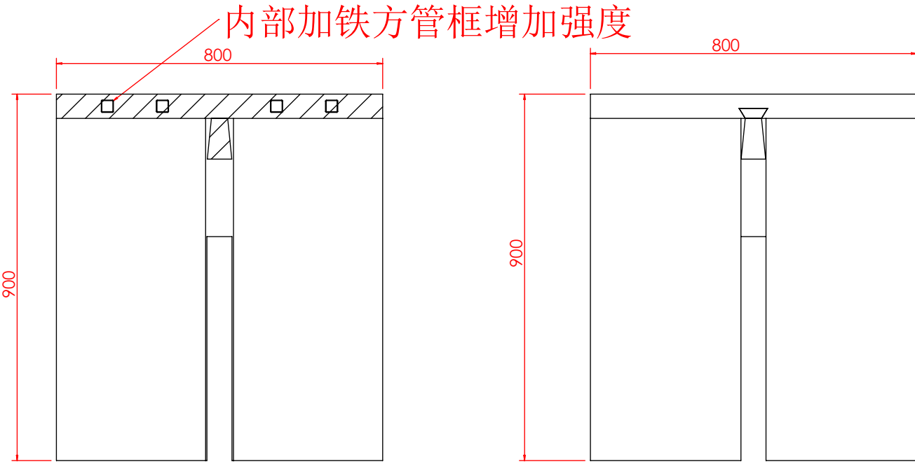
剖面 AG-AG
