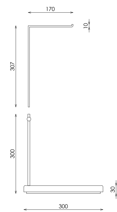
ALZADO
