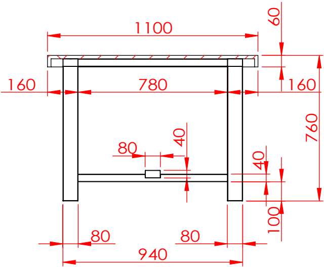
剖面 A-A
