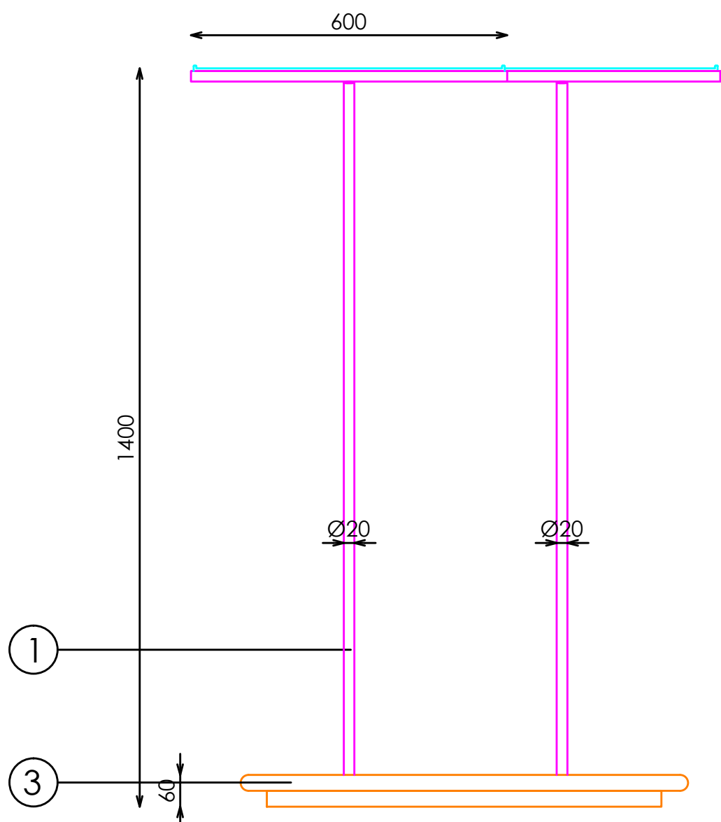
PERFIL IZQUIERDO
