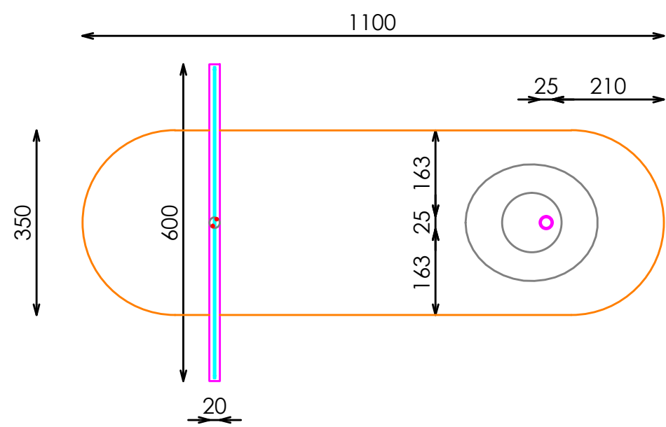
PLANTA
