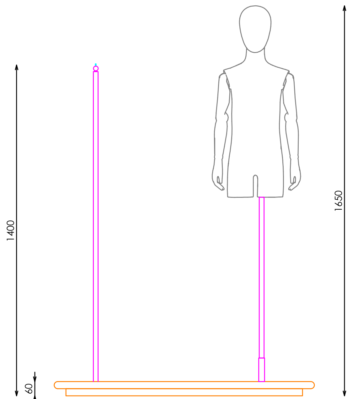
ALZADO
