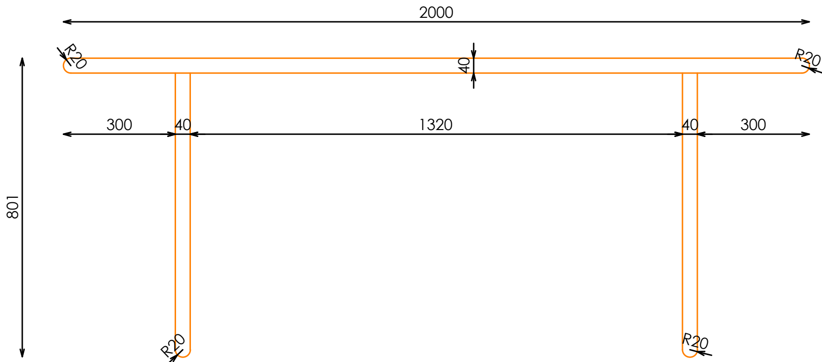
ALZADO
