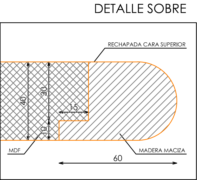
DETALLE SOBRE
