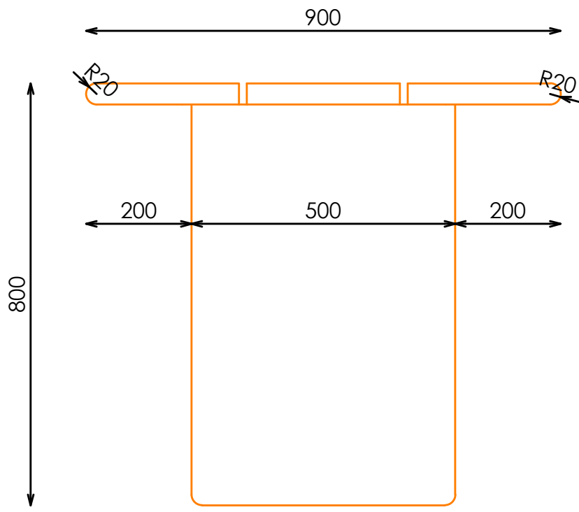
PERFIL
