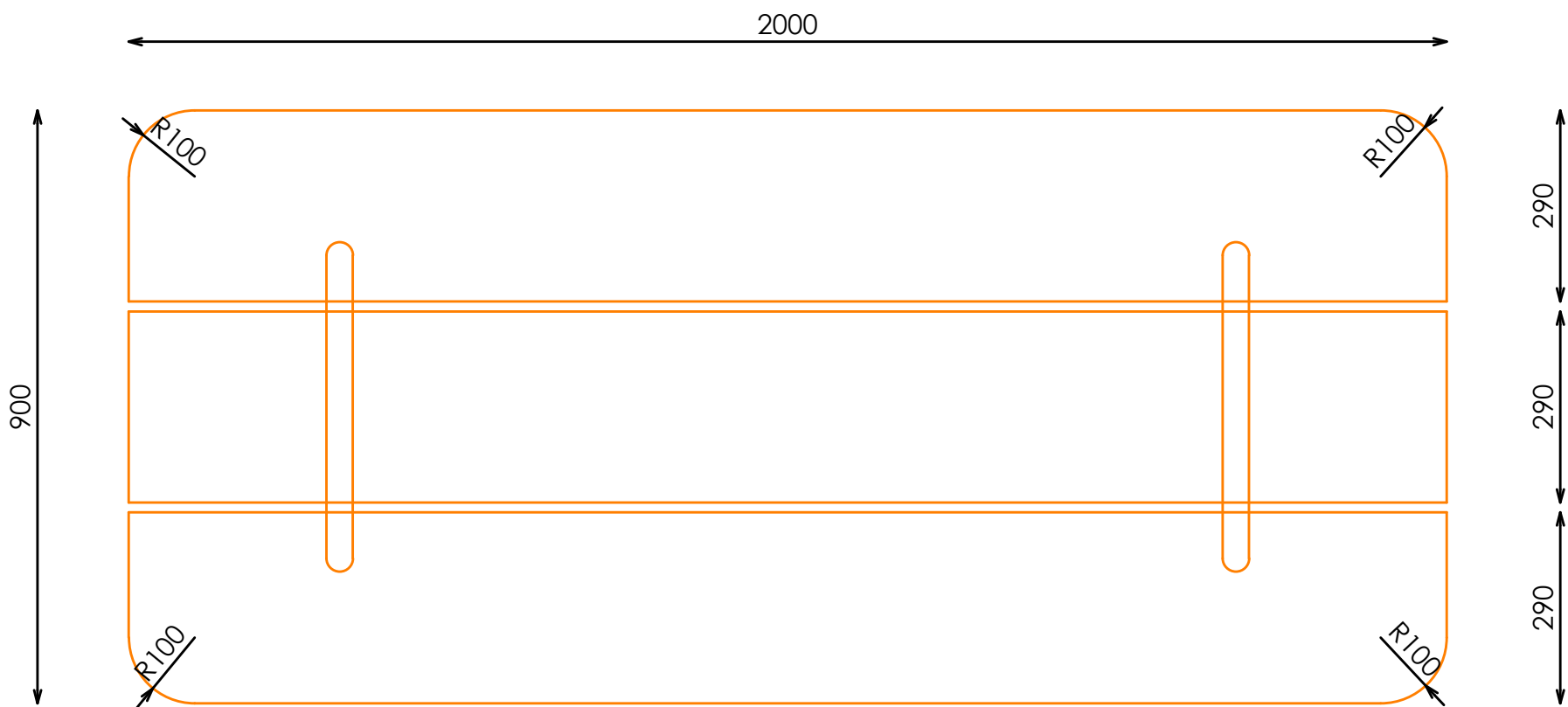
PLANTA
