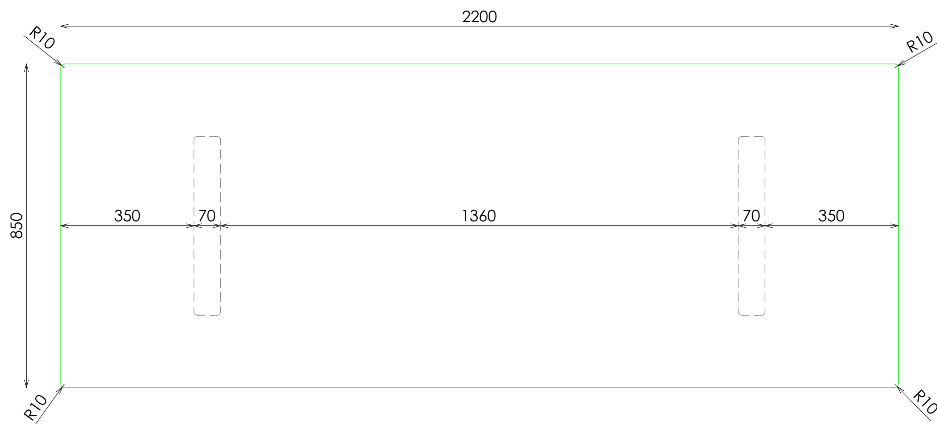
PLANTA
