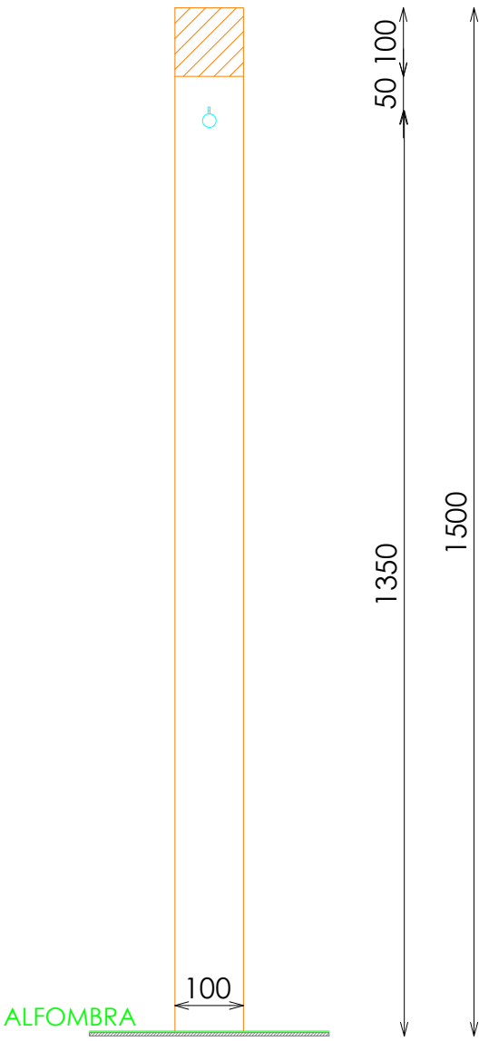
SECCION
