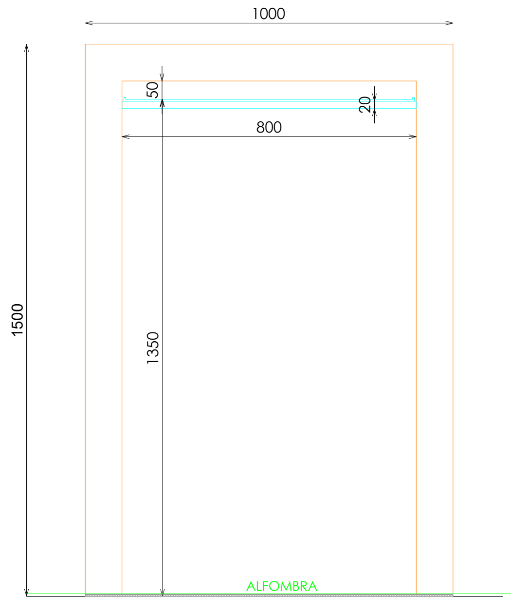
ALZADO
