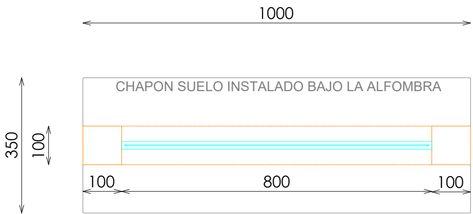
PLANTA
