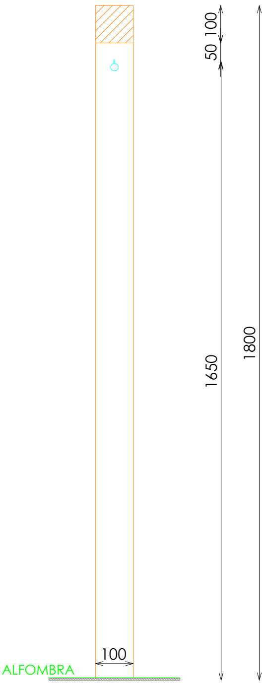
SECCION
