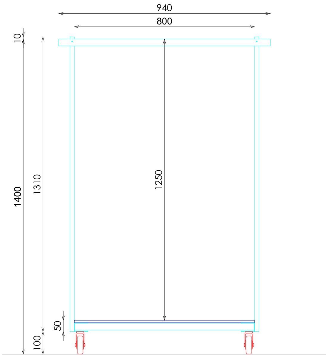
ALZADO SECCIONADO
