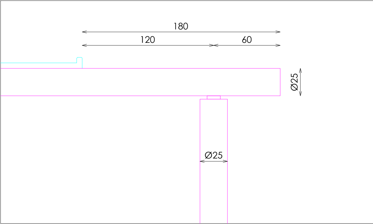
DETALLE A
