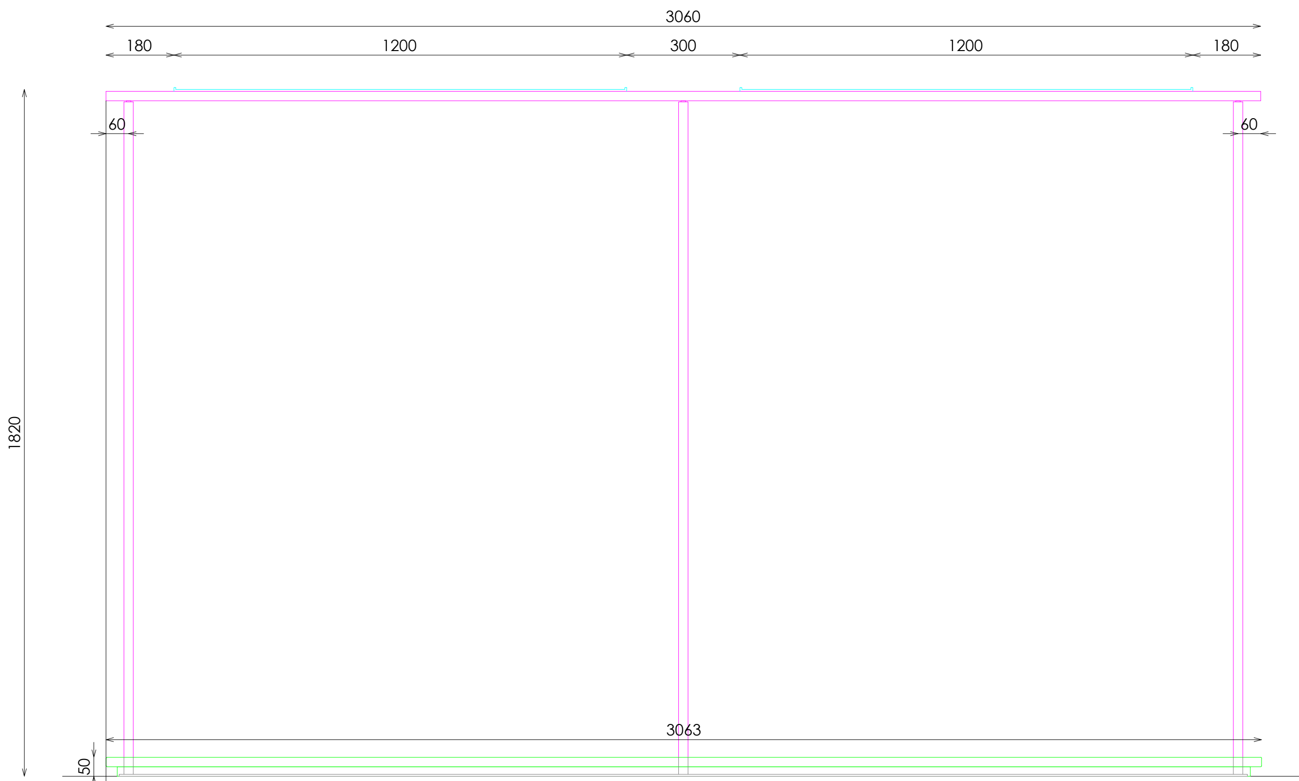
ALZADO
