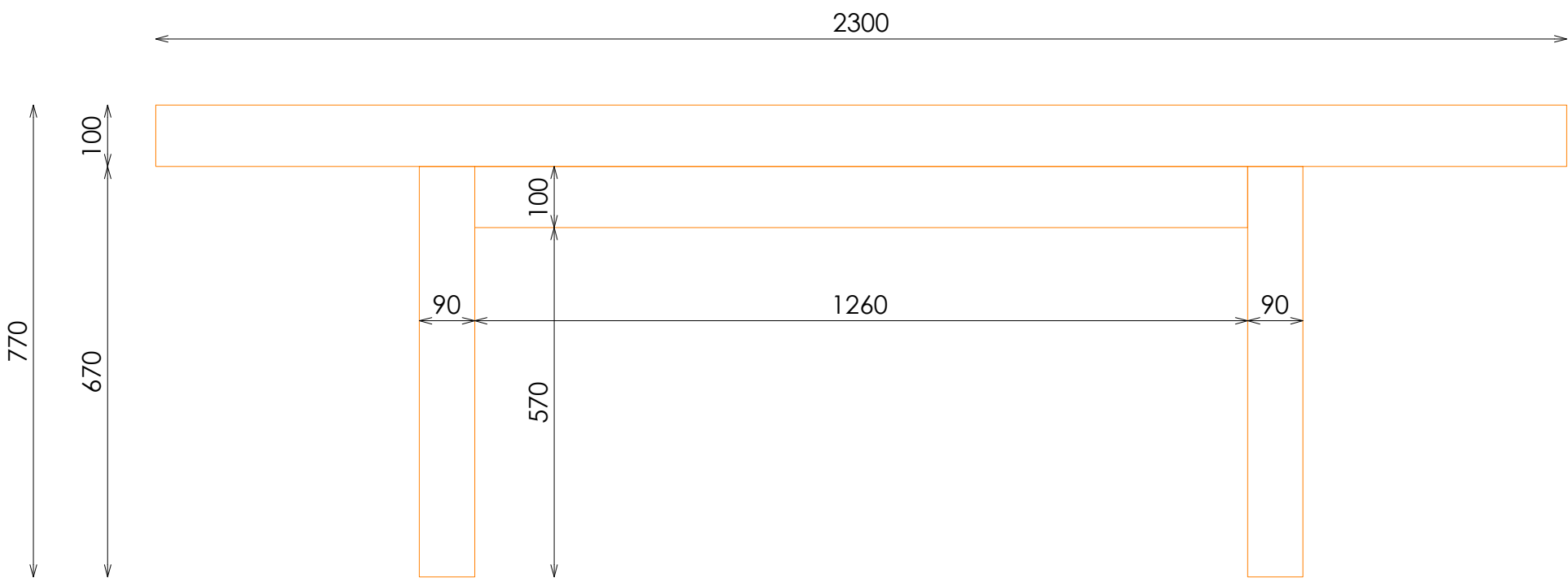
ALZADO FRONTAL
