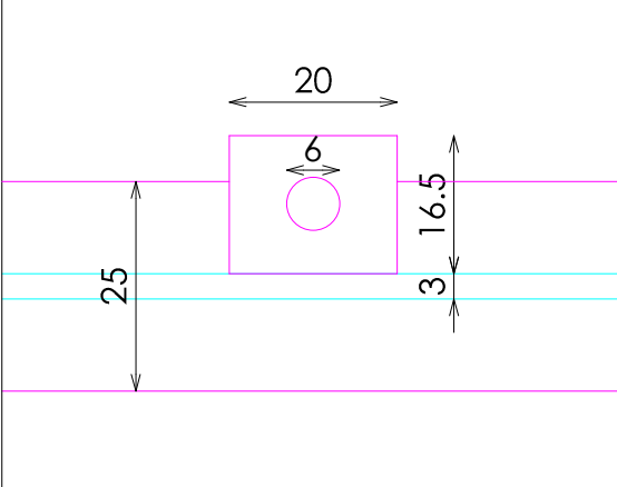
DETALLE ANCLAJE FRONTALES EXTRAIBLES
