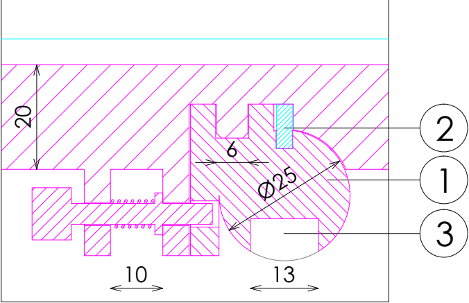
DETALLE ANCLAJE FRONTALES EXTRAIBLES
