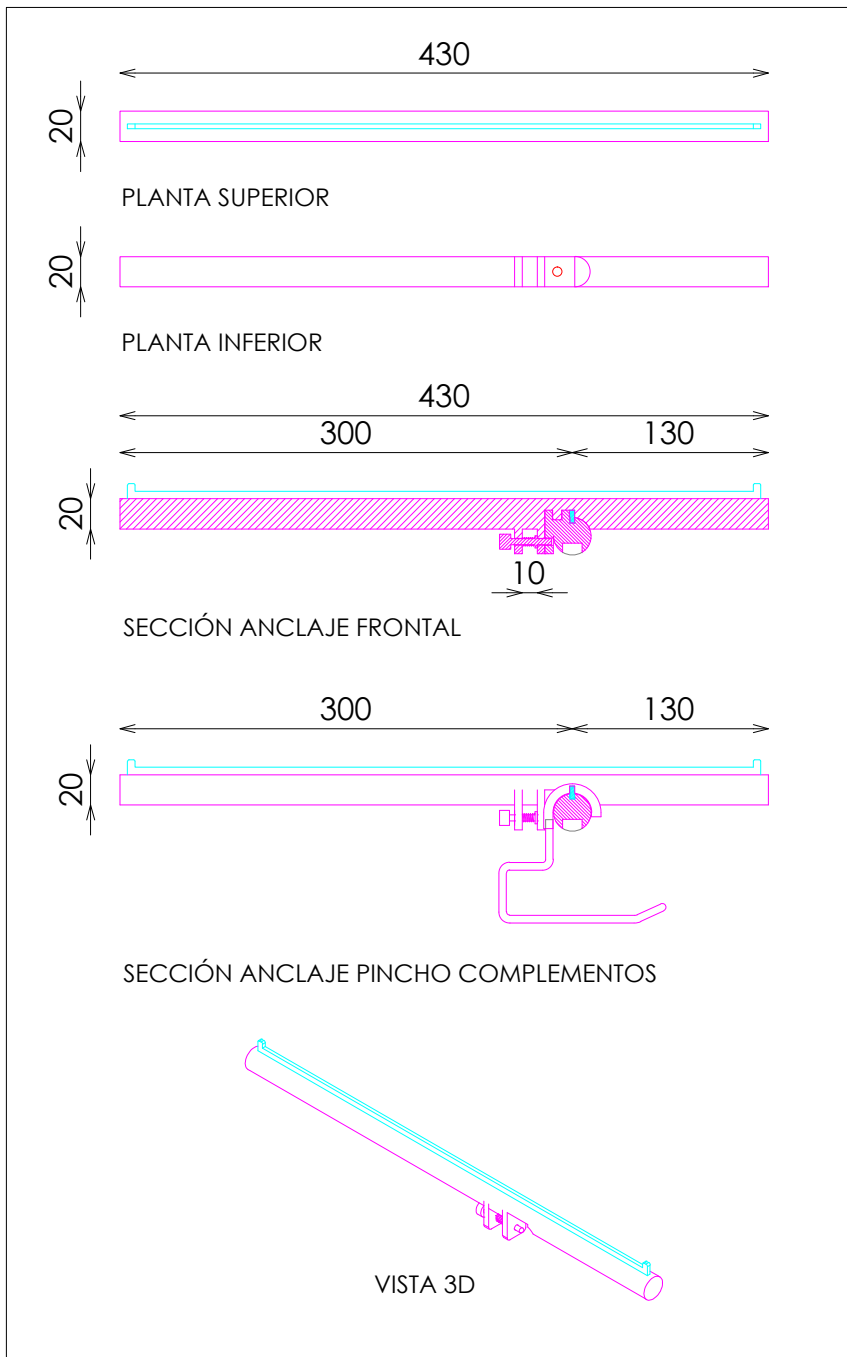
FRONTAL EXTRAIBLE
