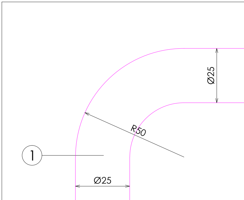
DETALLE A (ESQUINA BARRA)
