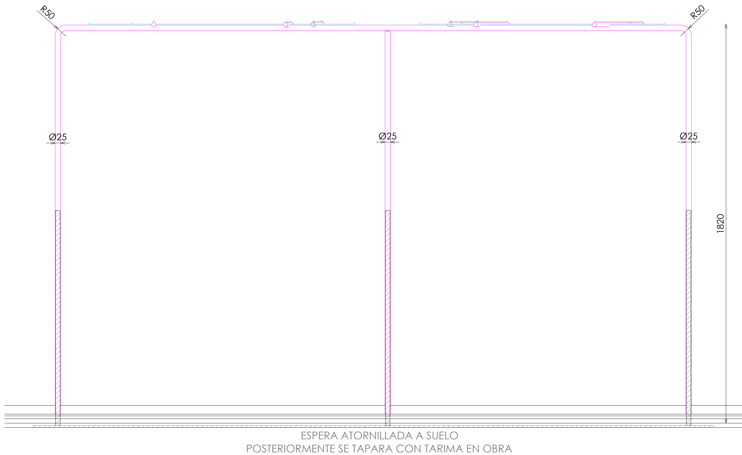
ALZADO FRONTAL
