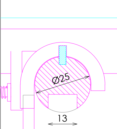
DETALLE BARRA ANCLAJE FRONTALES
