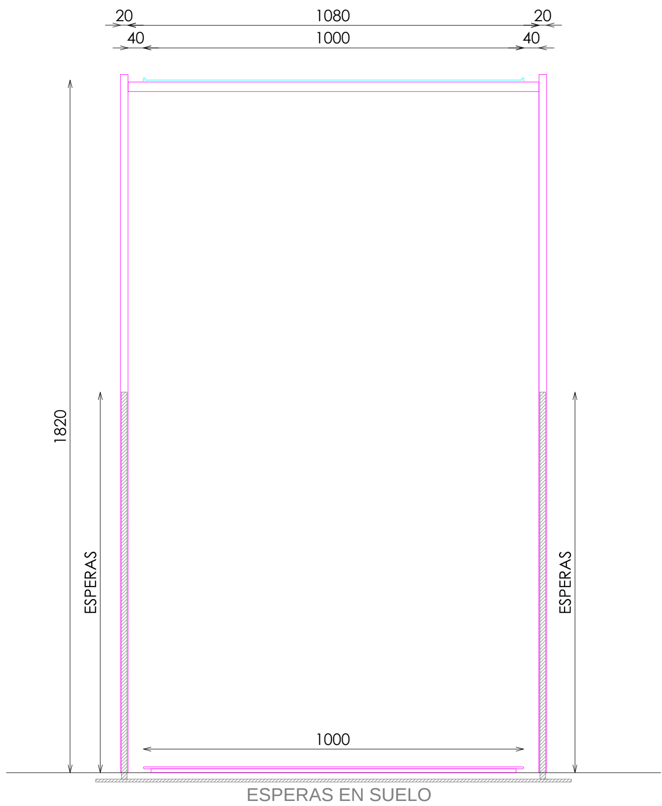
ALZADO SECCIONADO
