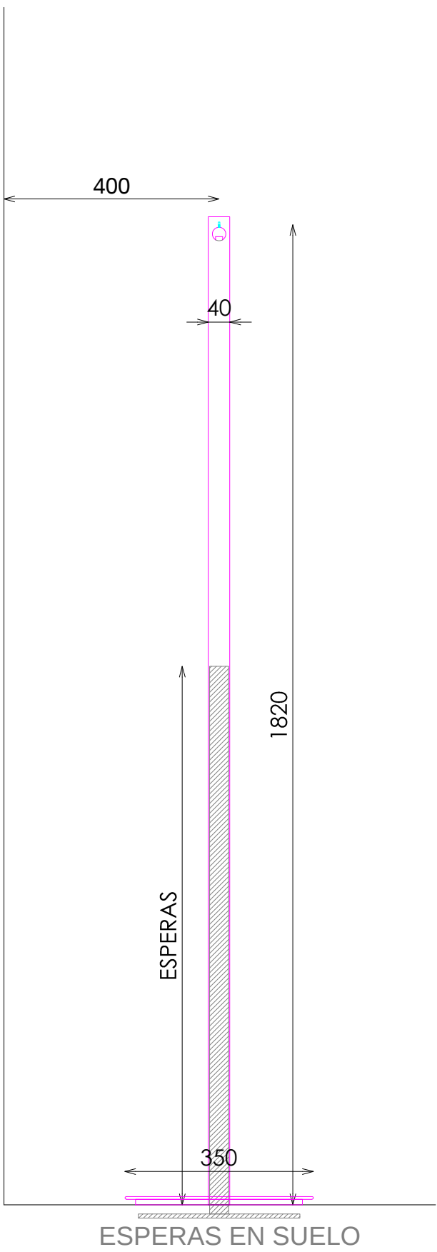
PERFIL SECCIONADO
