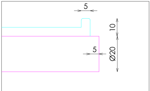
DETALLE ANTIROCE
