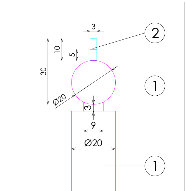
DETALLE ANTIROCE
