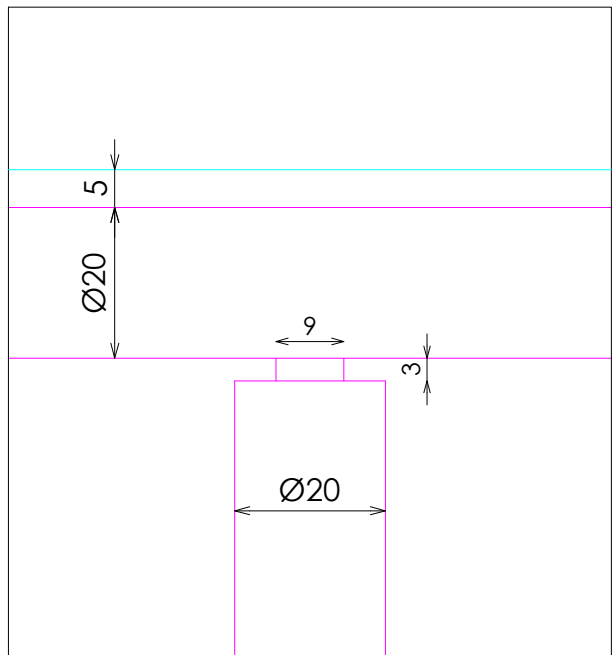
DETALLE C
