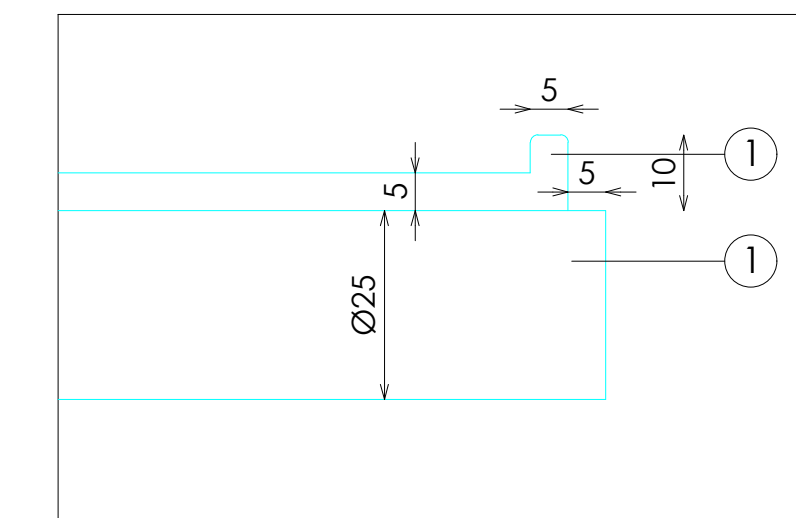
DETALLE C
