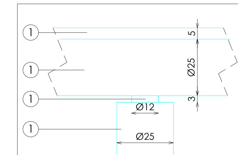
DETALLE B
