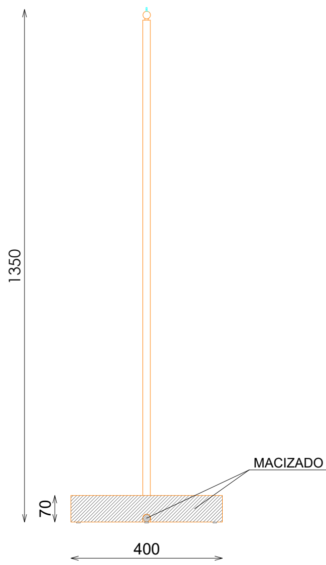
PERFIL
