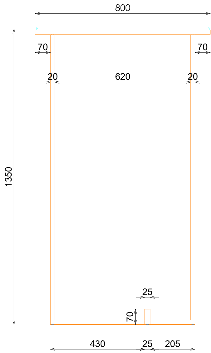
ALZADO
