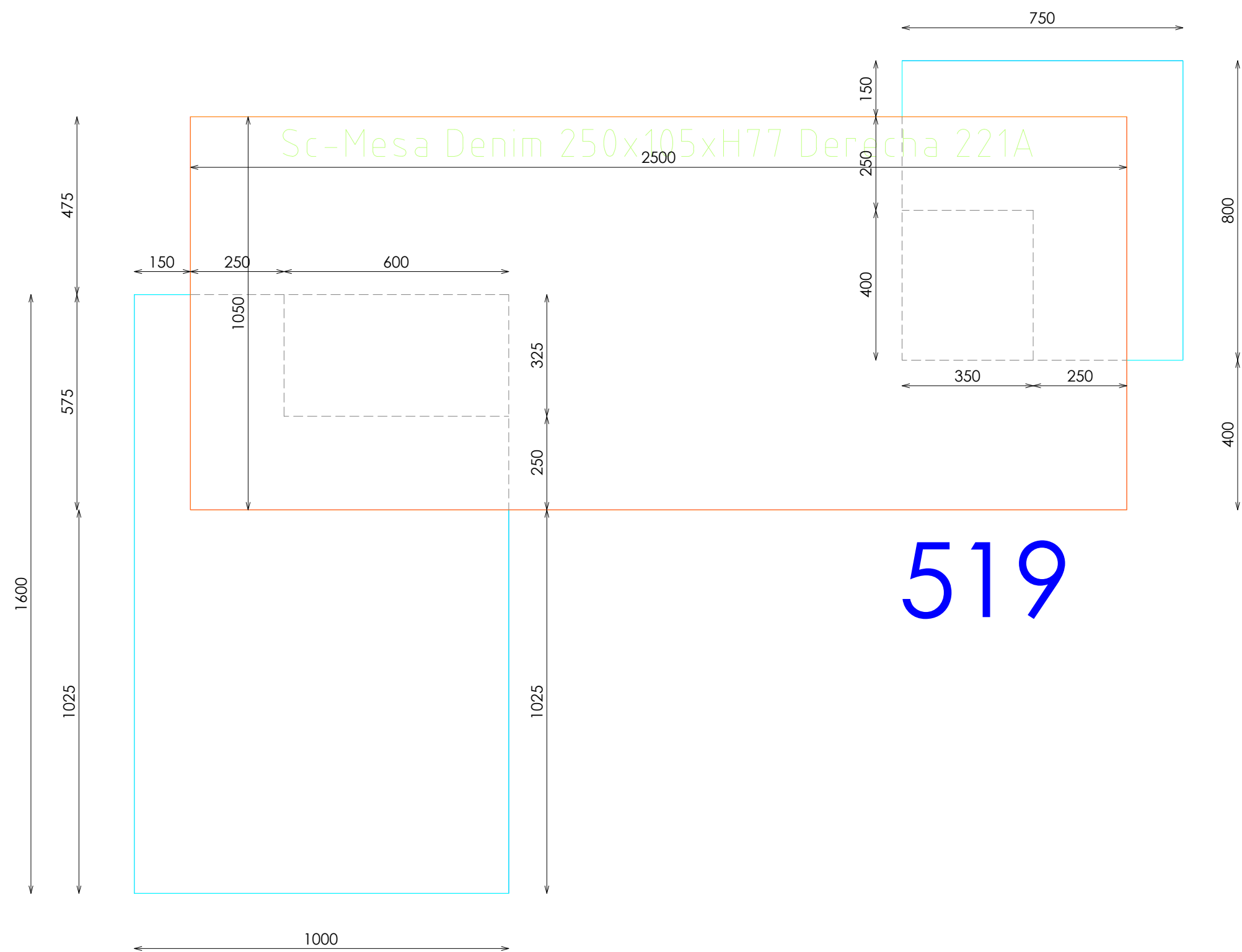
PLANTA
