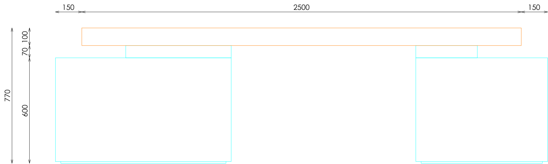
ALZADO FRONTAL
