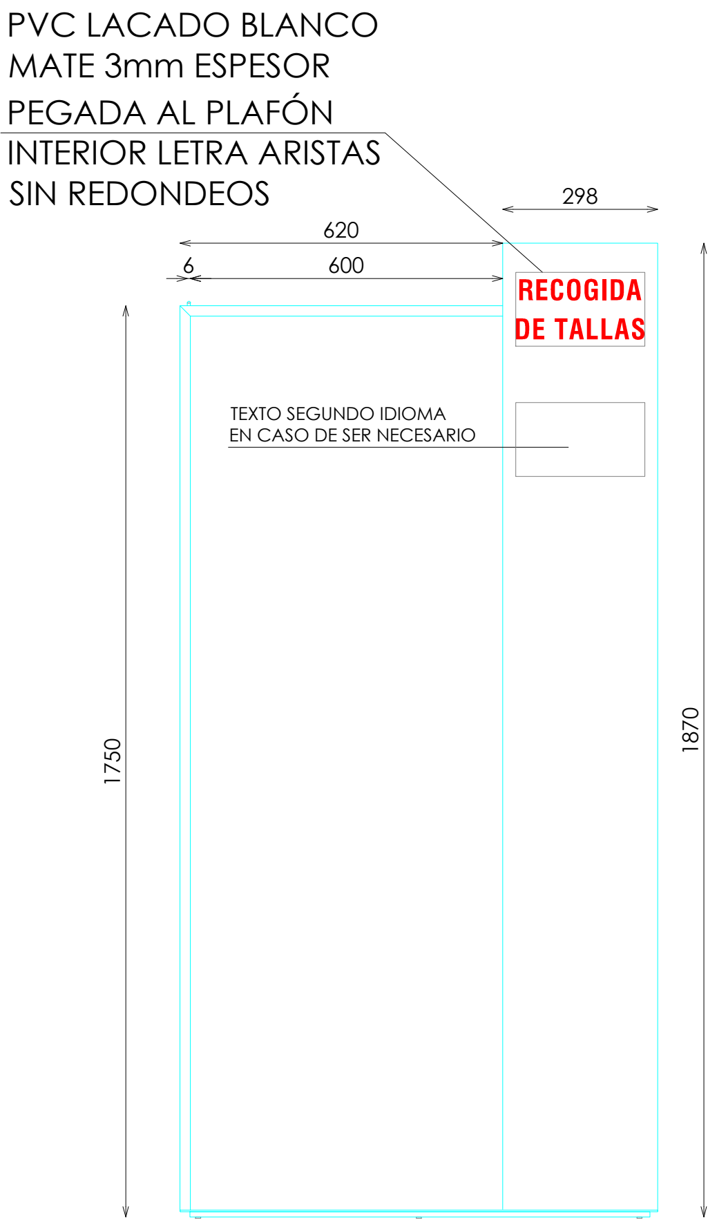
ALZADO POSTERIOR
