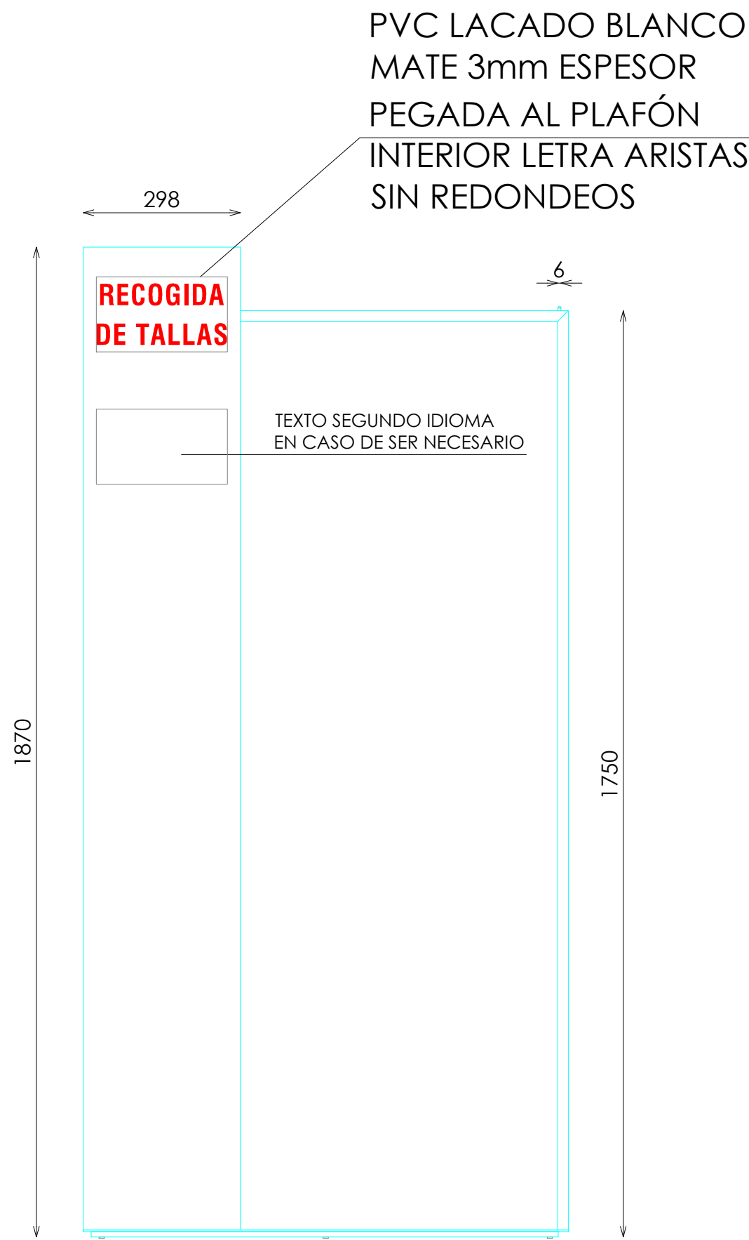
ALZADO FRONTAL
