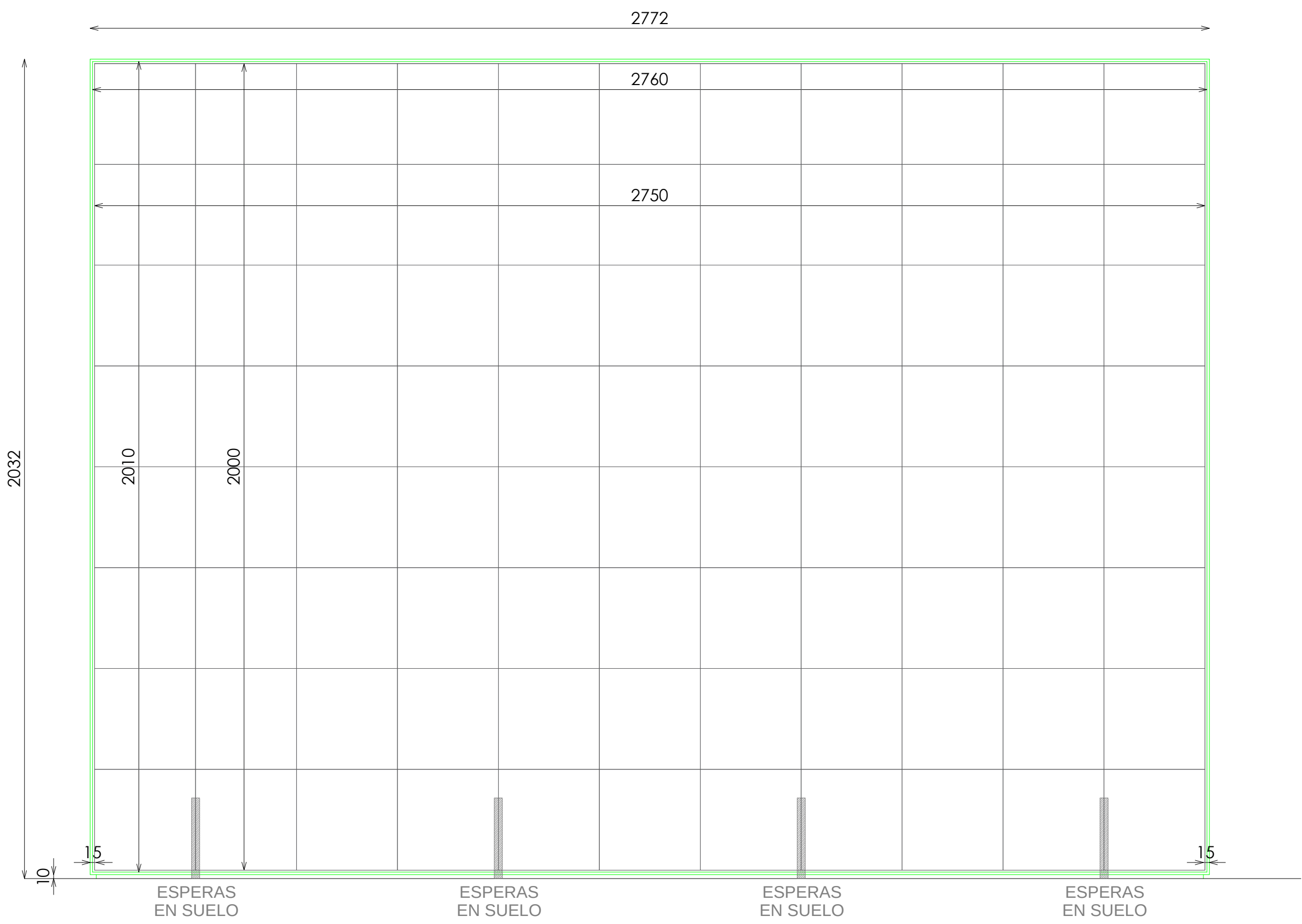
ALZADO
