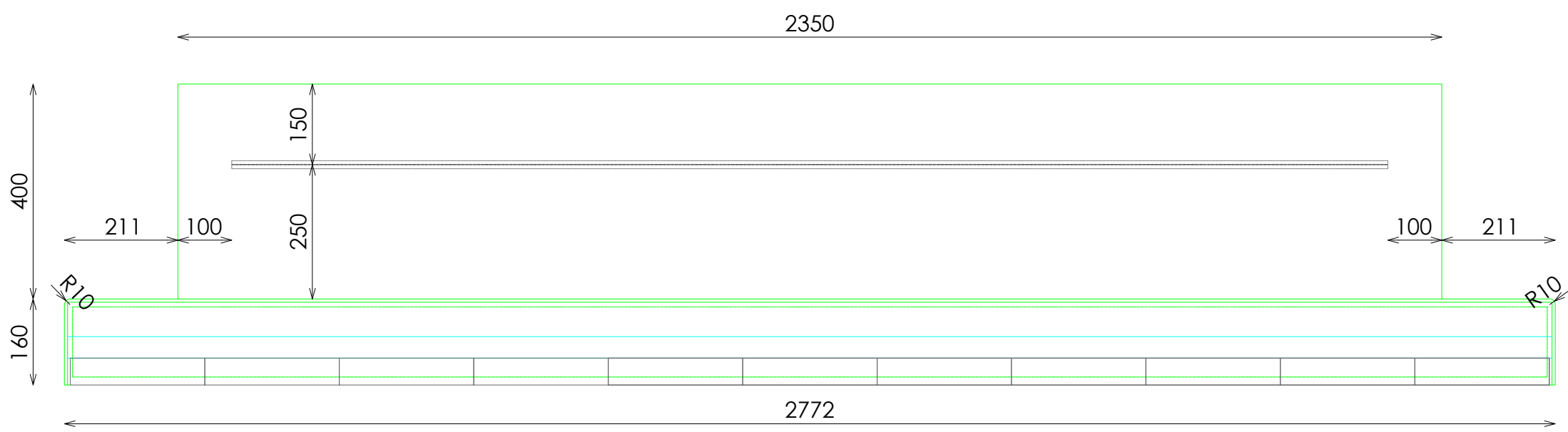
PLANTA
