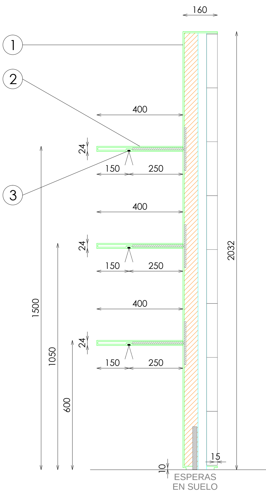
SECCION
