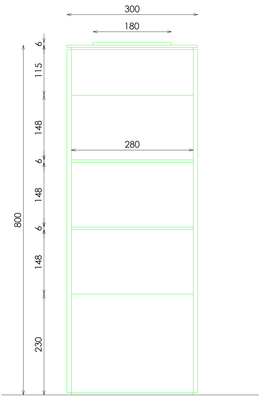
ALZADO FRONTAL
