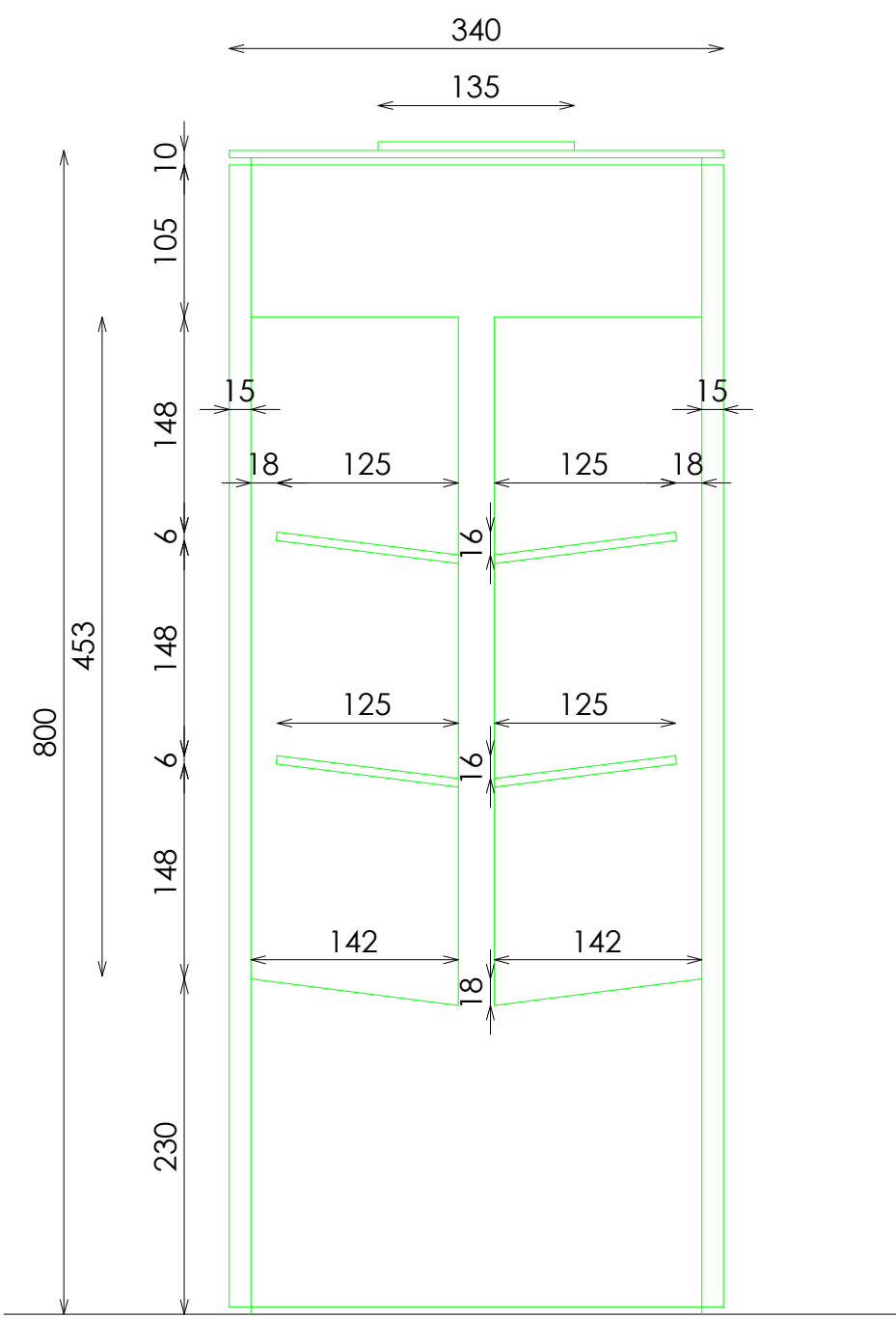
SECCION
