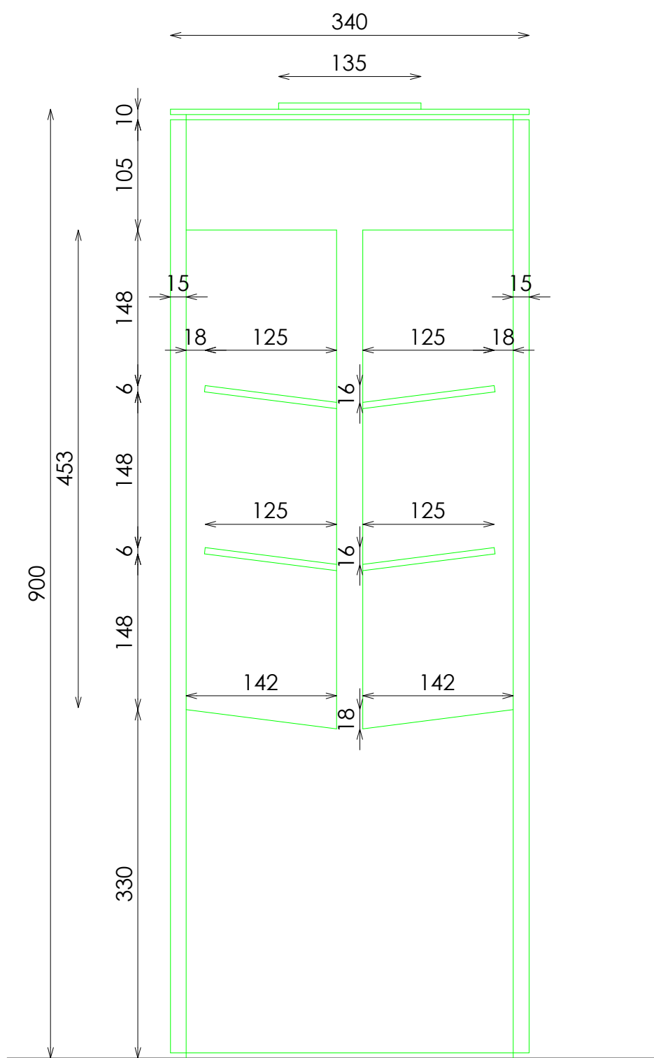
SECCION
