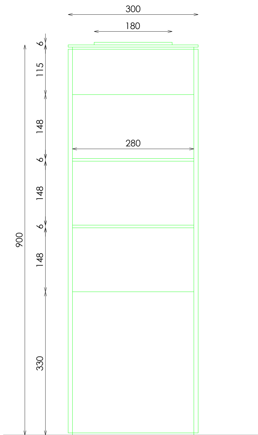
ALZADO FRONTAL
