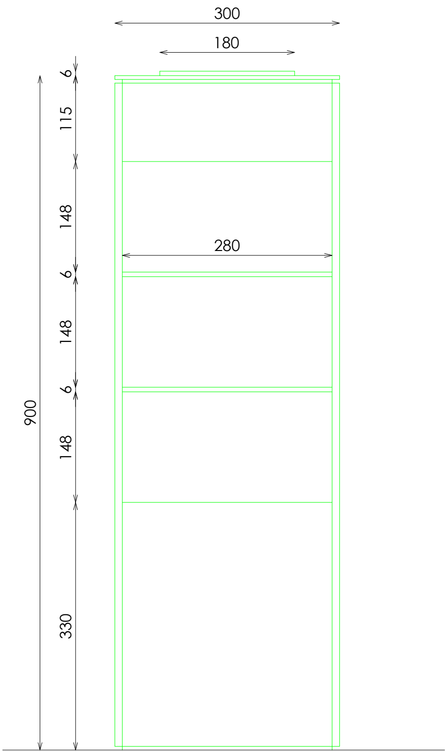
ALZADO FRONTAL
