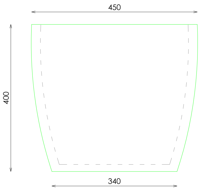
ALZADO FRONTAL
