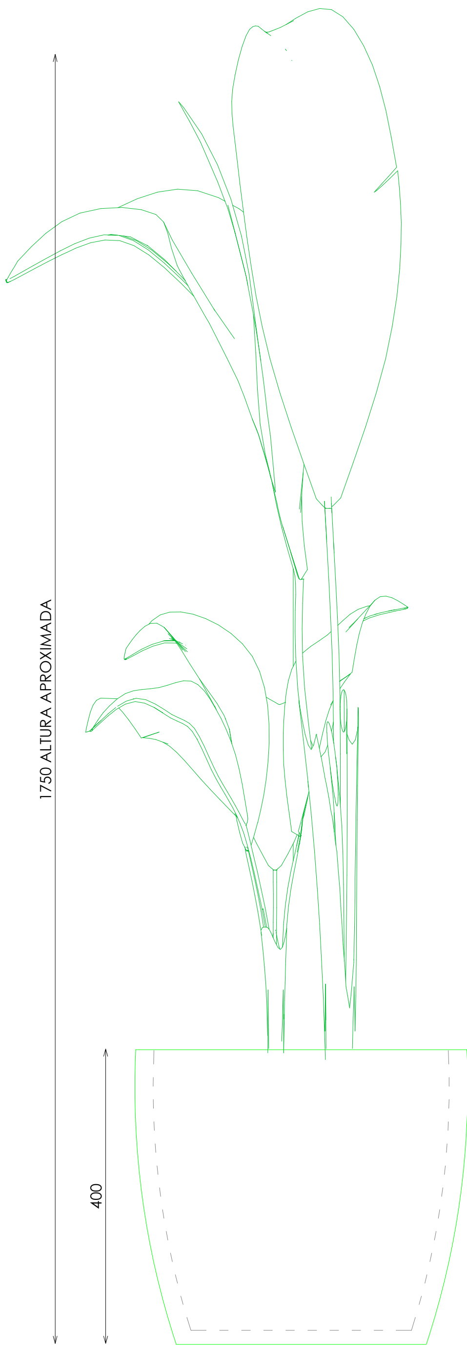
EJEMPLO ALZADO MACETERO+PLANTA
