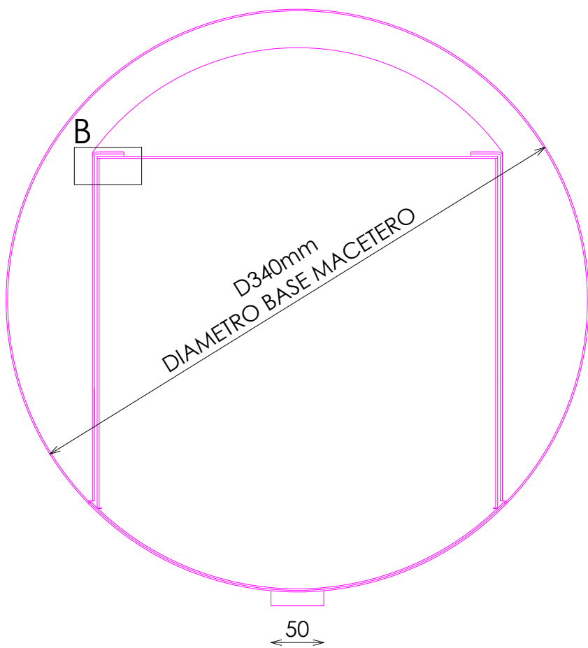
PLANTA SECCIONADA
