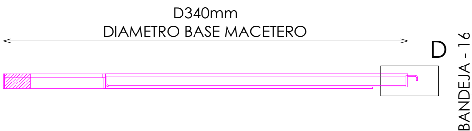
PERFIL SECCIONADO
