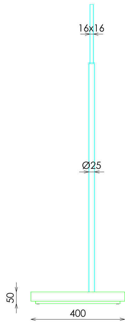
ALZADO (SIN BUSTO)
