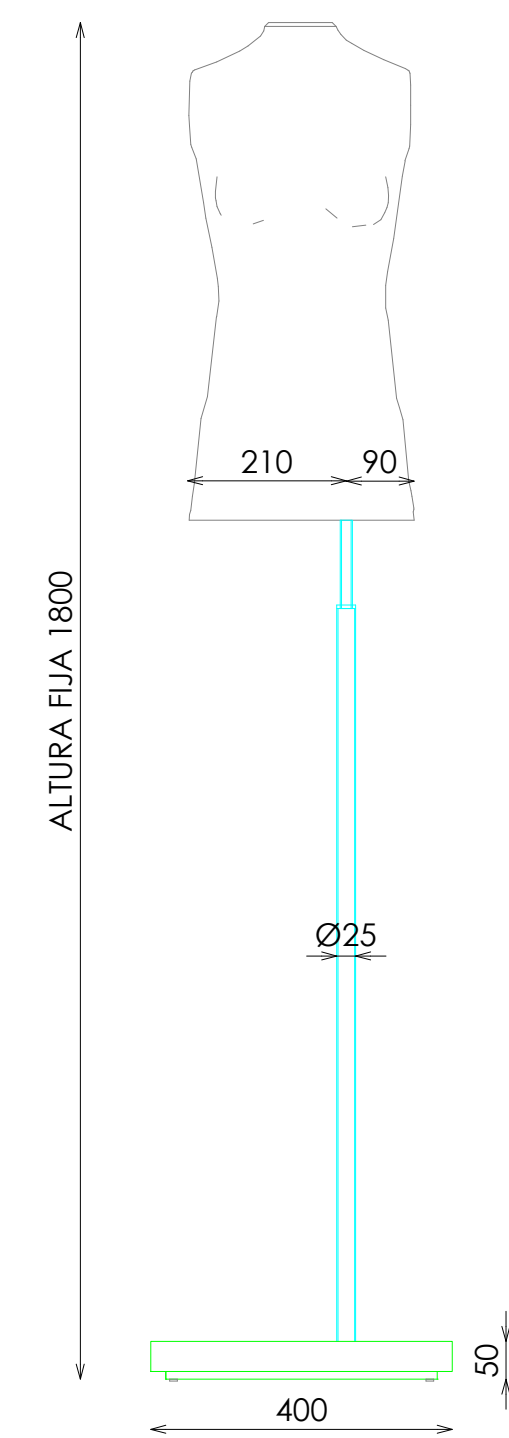
ALZADO
