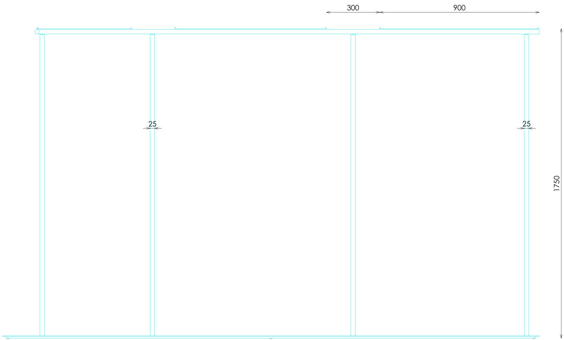
ALZADO
