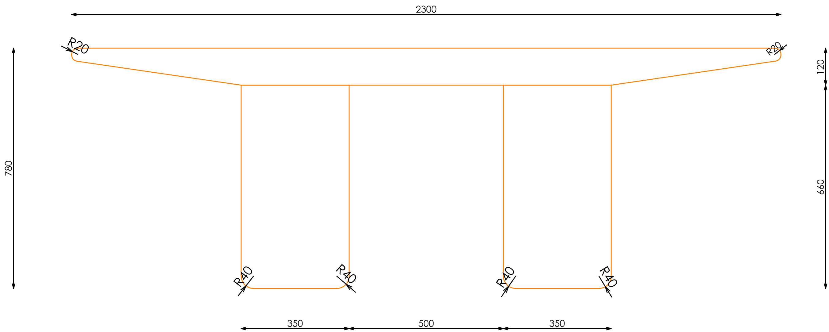
ALZADO FRONTAL
