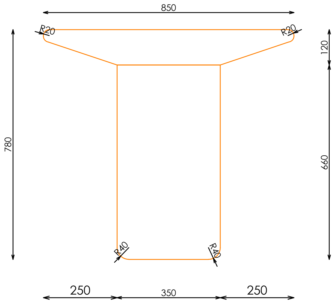
ALZADO LATERAL
