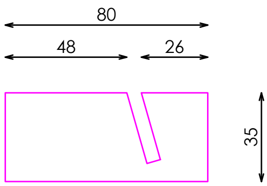
SECCIÓN
