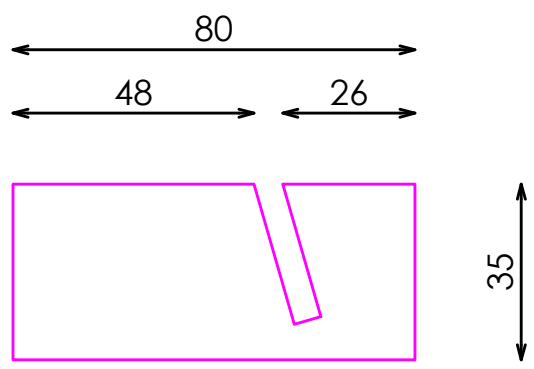
SECCIÓN
