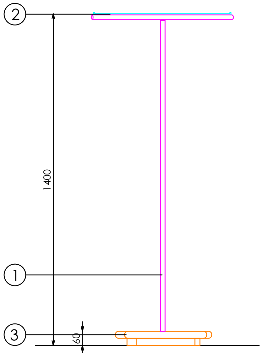
ALZADO LATERAL
