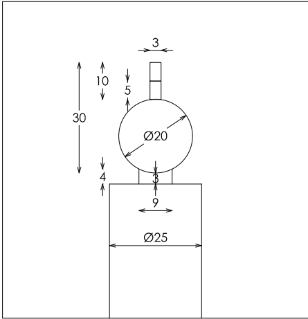
DETALLE B
