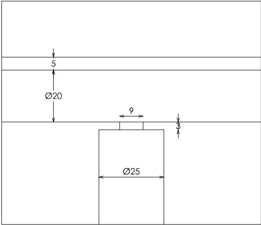
DETALLE A
