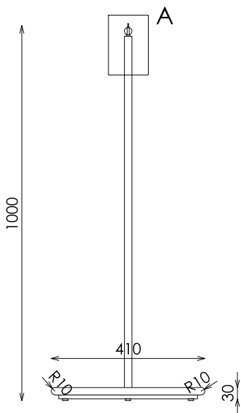
PERFIL
