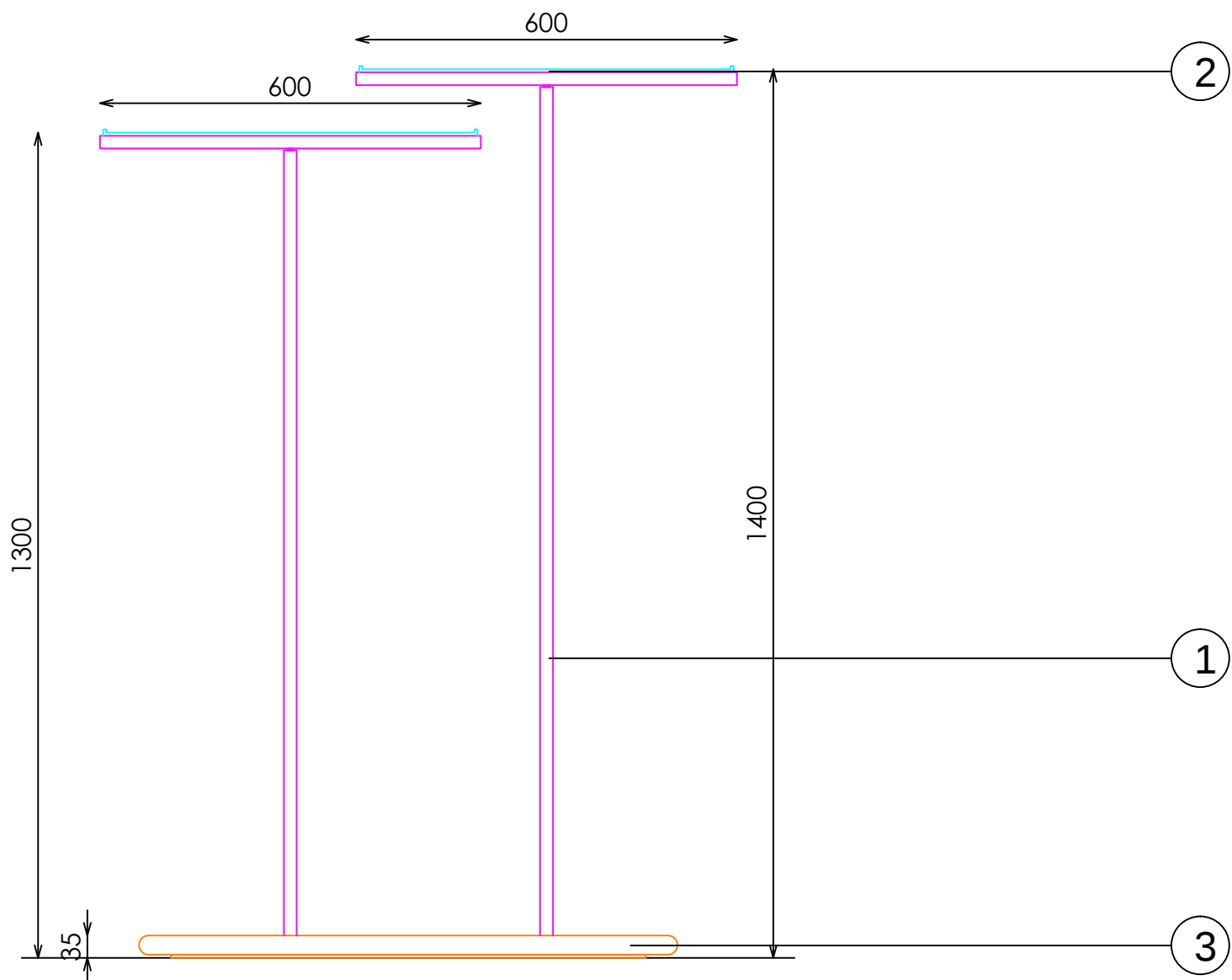
ALZADO LATERAL
