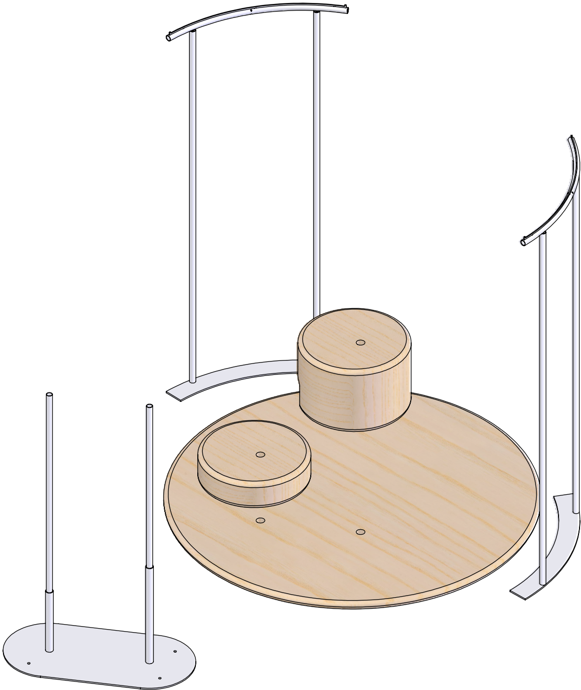
爆炸图
