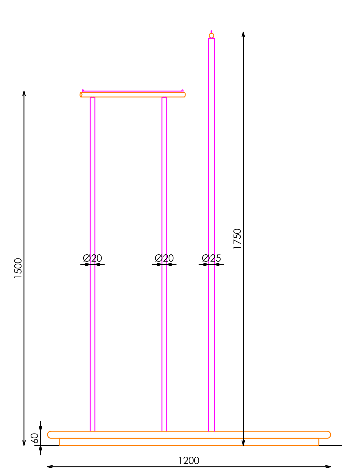
ALZADO FRONTAL
