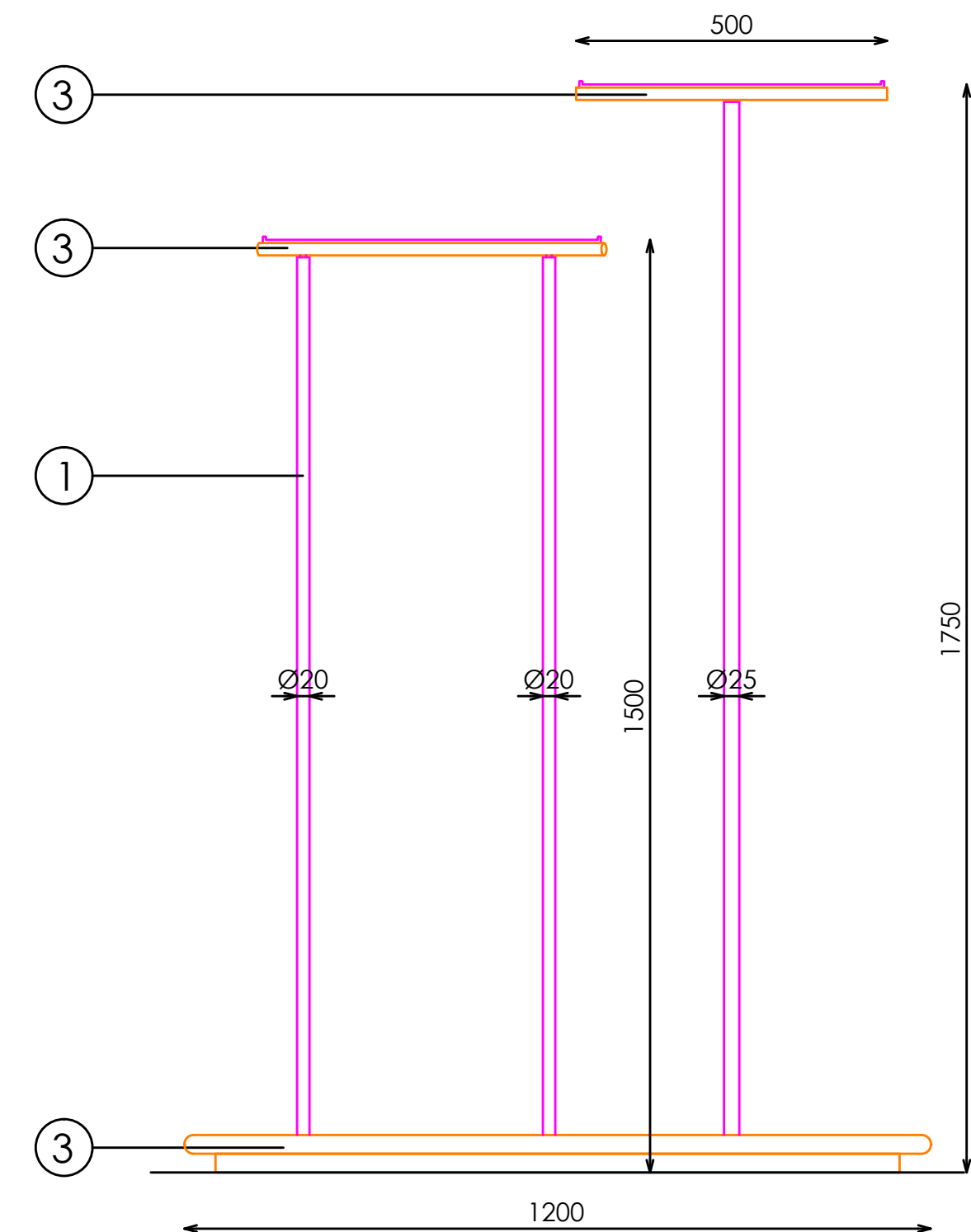
ALZADO LATERAL IZQUIERDO (VISTA FRONTAL COLLET)
