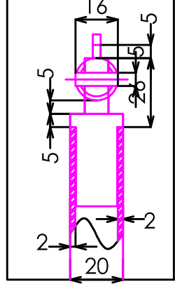
DETALLE B
