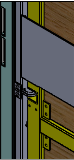
局部视图 AJ 比例 1:5 -总装
