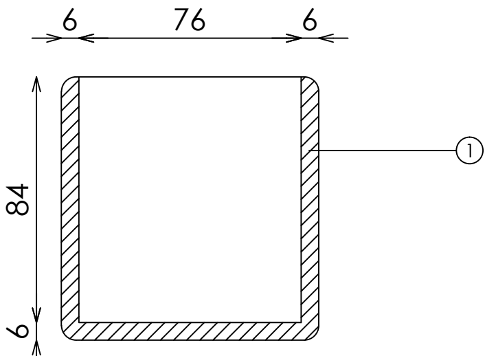
PERFIL SECCIONADO
