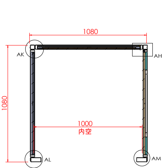
剖面 AG-AG
