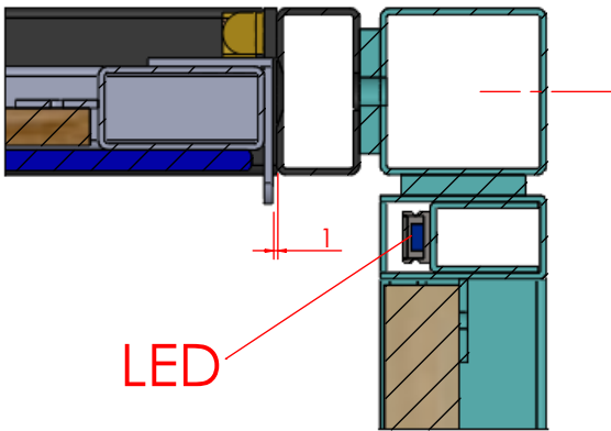
局部视图 AH 比例 1 : 2
