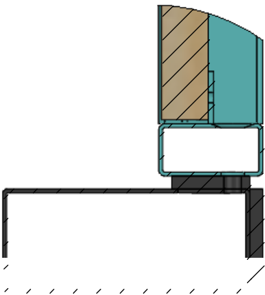
局部视图 AM 比例 1 : 2
