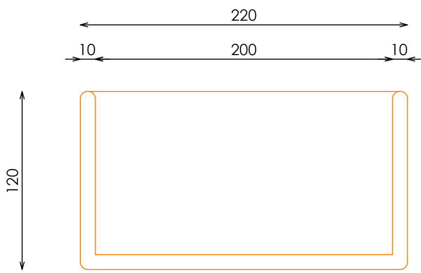
PERFIL
