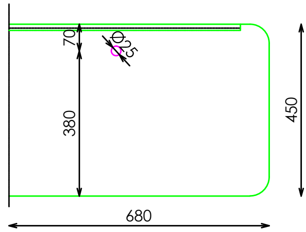
PLANTA SECCIONADA (ILUMINACIÓN EN TARIMA)
