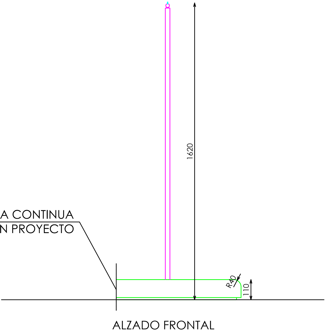
ALZADO FRONTAL
