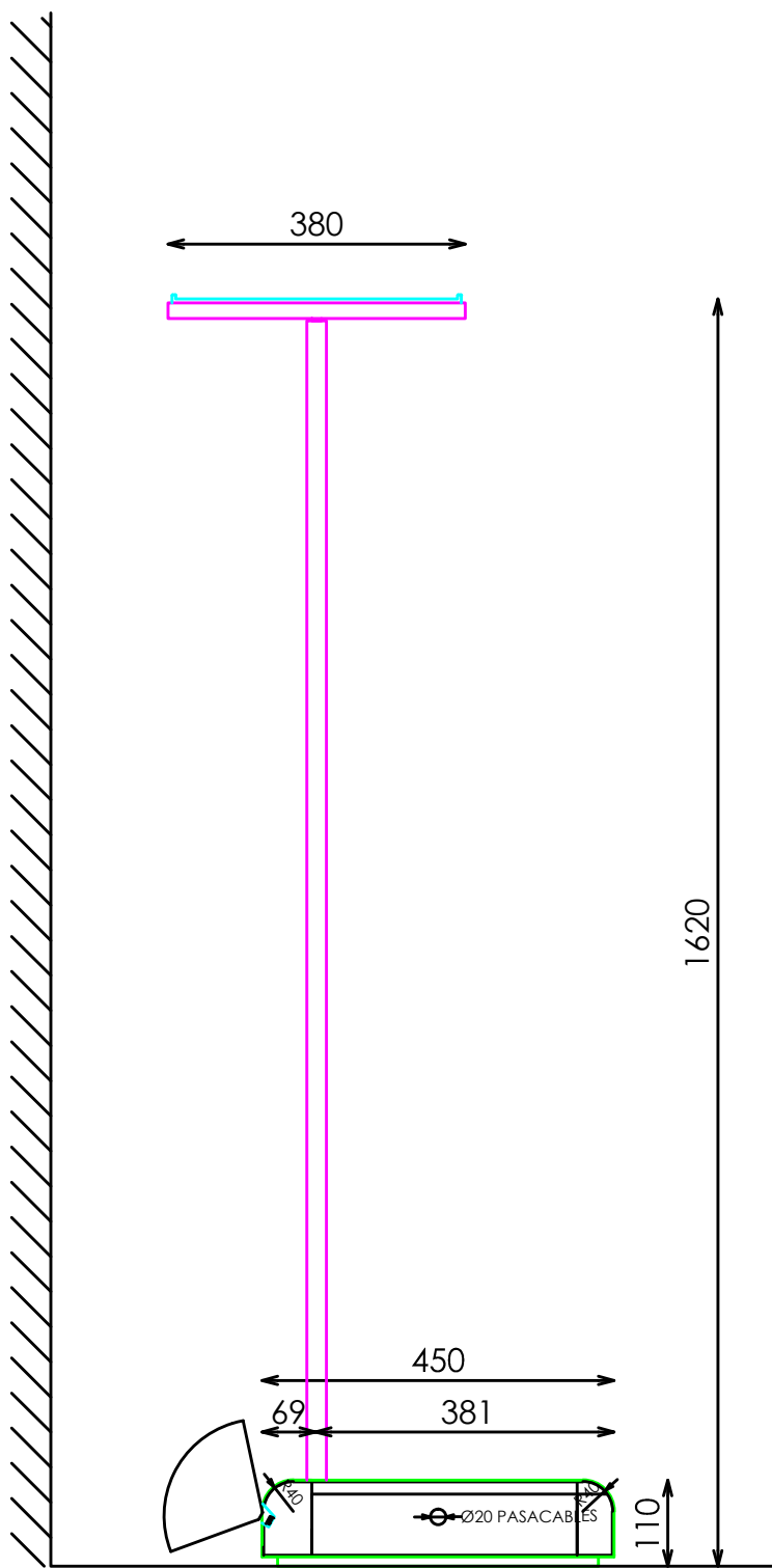
PERFIL SECCIONADO
