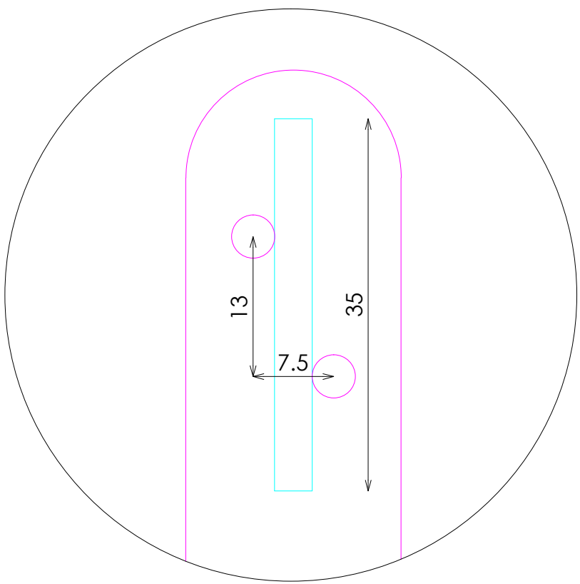
DETALLE A
