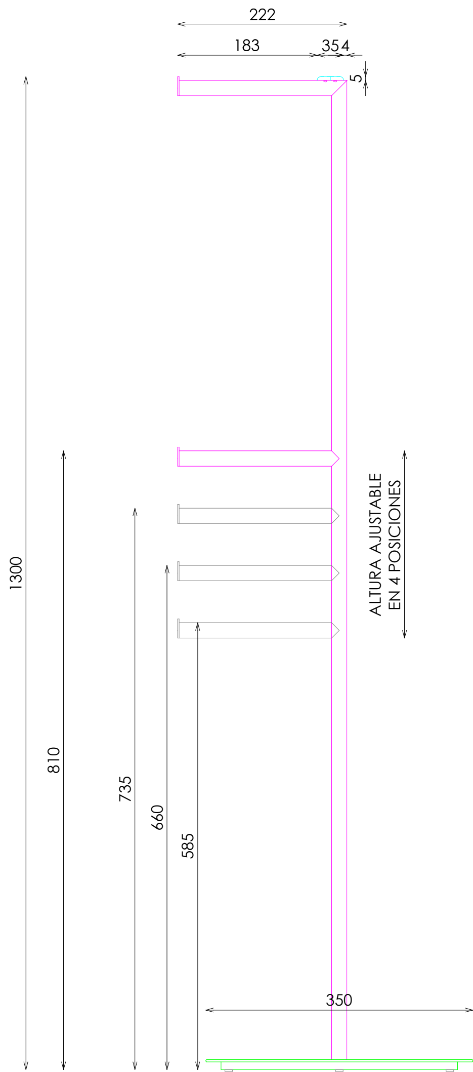
ALZADO
