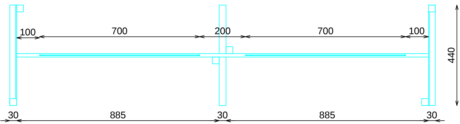
PLANTA
