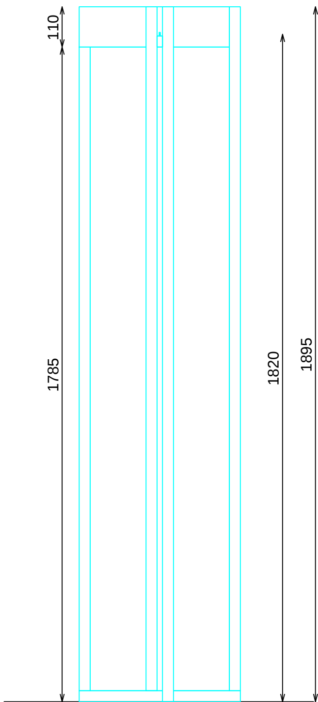
SECCION
