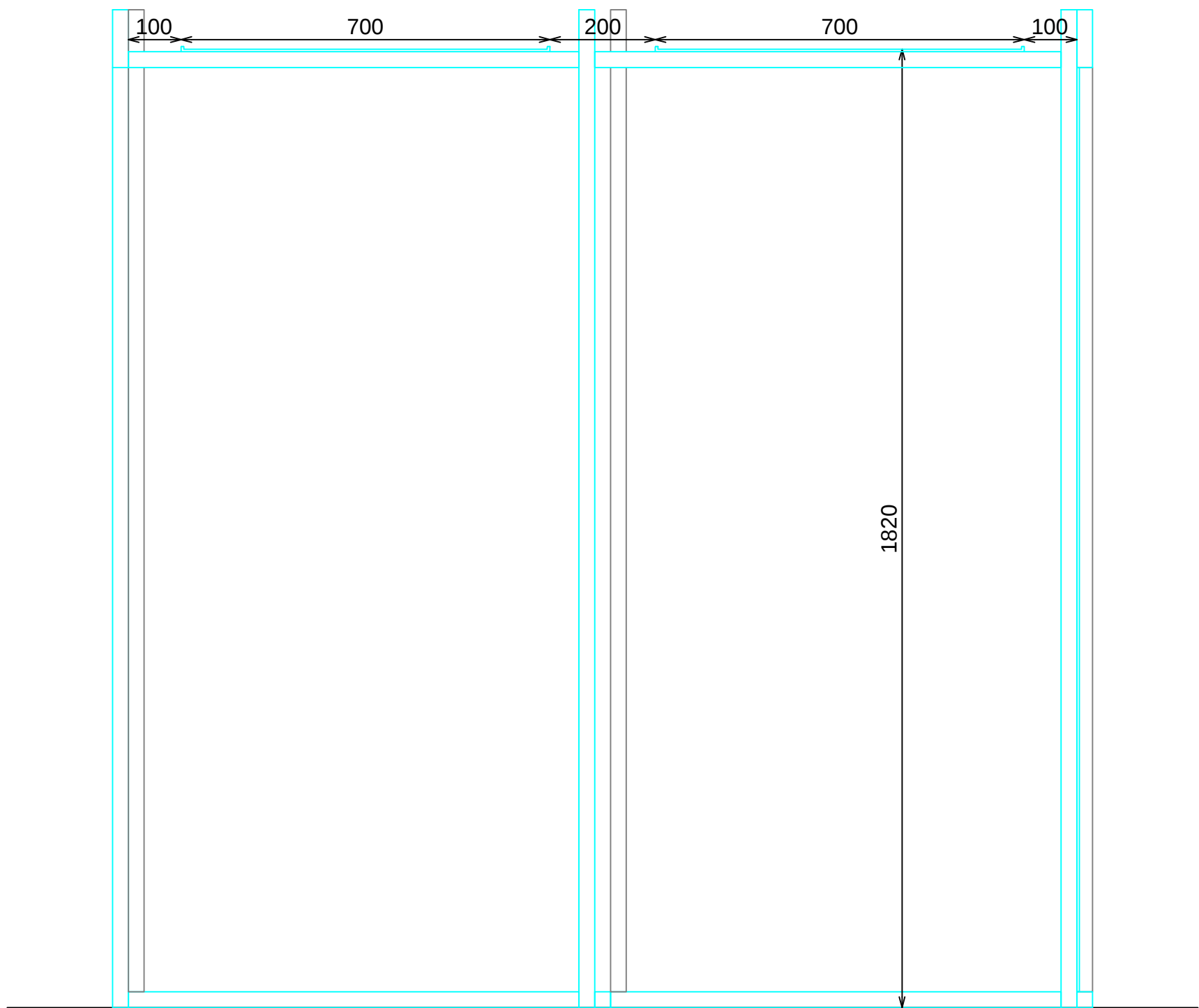
ALZADO FRONTAL
