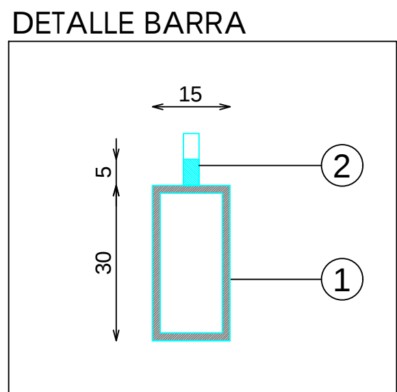
DETALLE BARRA
