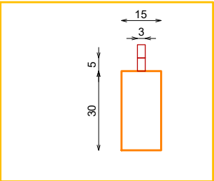
DETALLE BARRA
