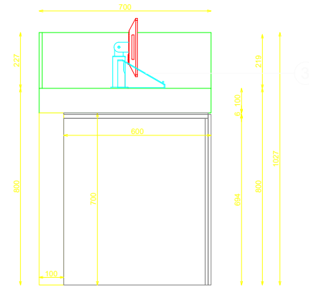
PERFIL
